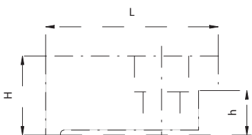
Прижим для 6586
